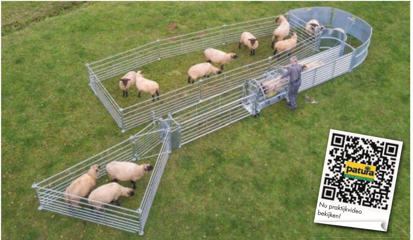
Complete installatie voor het vangen, behandelen en sorteren van schapen.
