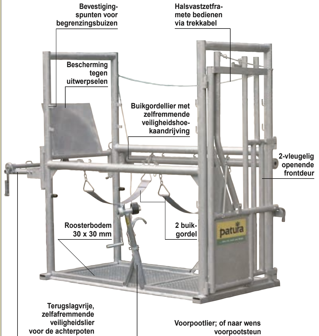
Comfortabele voorpootlier voor het gemakkelijk opheffen van de voorpoten
