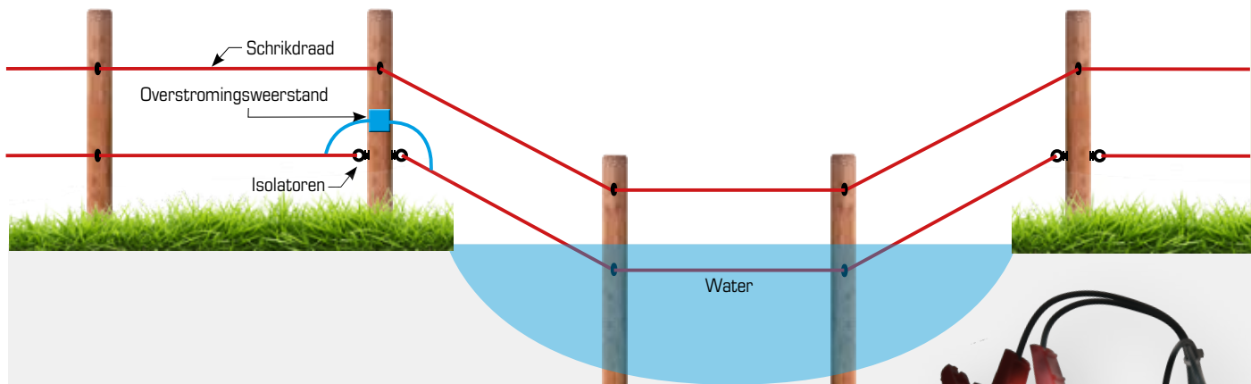
8. OVERSTROMINGS EN AANGROEI BESCHERMER Hiermee beschermt u uw hoofdafastering tegen verwachte, maar niet te vermijden kortsluiting door overstroming en/of zware aangroei.
